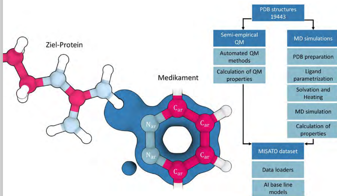
Abbildung 3: Das Konzept des MISATO-Datensatzes. Das Biomolekül (links) wird durch ein atomistisches, dynamisches Modell dargestellt. Das Arzneimittelmolekül wird durch seine vollständige elektronische Darstellung dargestellt, die aus quantenchemischen Berechnungen stammt. Die komplette Kuratierung und Bereitstellung des Datensatzes ist für einen einfachen Zugang optimiert. (Quelle: Grzegorz Popowicz).
