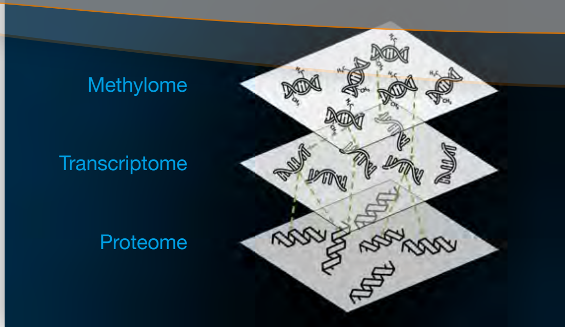
Abbildung 2: Modelhafte Darstellung einer Multi-omics Analyse von DNA-Methylierung (Methylome), Genexpression (Transcriptome) und Proteinexpression (Proteome) (Quelle: basierend auf Argelaquet et al. (2018)).
